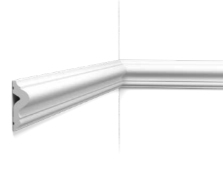
PX175 | PX175F Duropolymer® 200 x 5 x 1,7 cm
