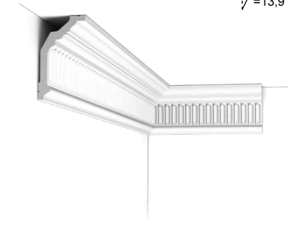
C304 | C304F Purotouch® 200 x 12,2 x 7,2 cm
